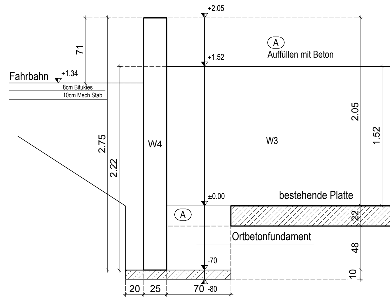
Schnitt 1
